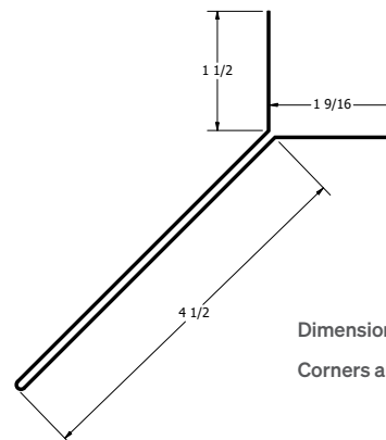
Y Fin External Corner Trim
